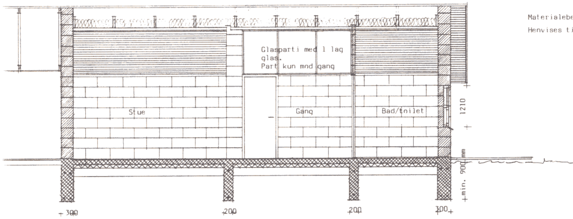
SNIT A-A MÅL 1:50
