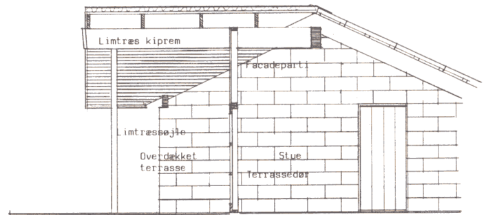
SNIT C-C MÅL 1:50
