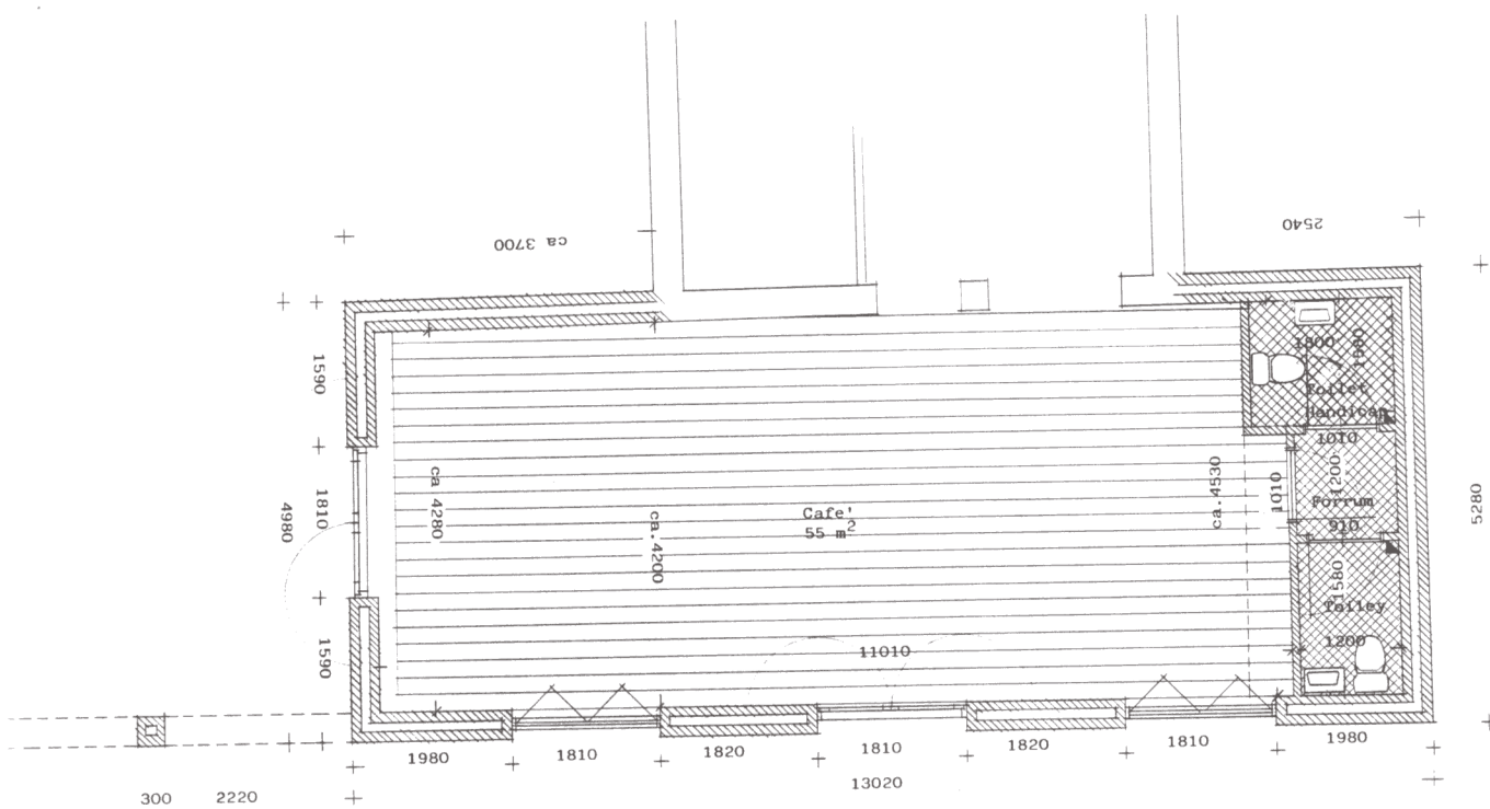
Grundplan mål 1:50 ( udvidelse )
